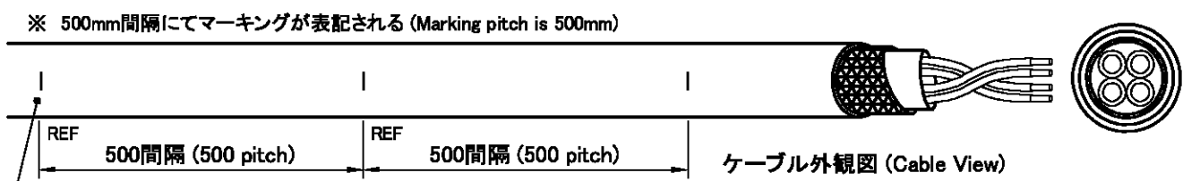
構造図・コア識別 (Structure & Core Distinction)
